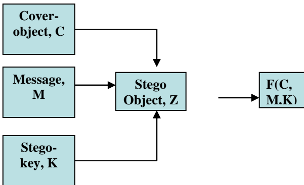
الشكل (3:5): مكونات Steganography
